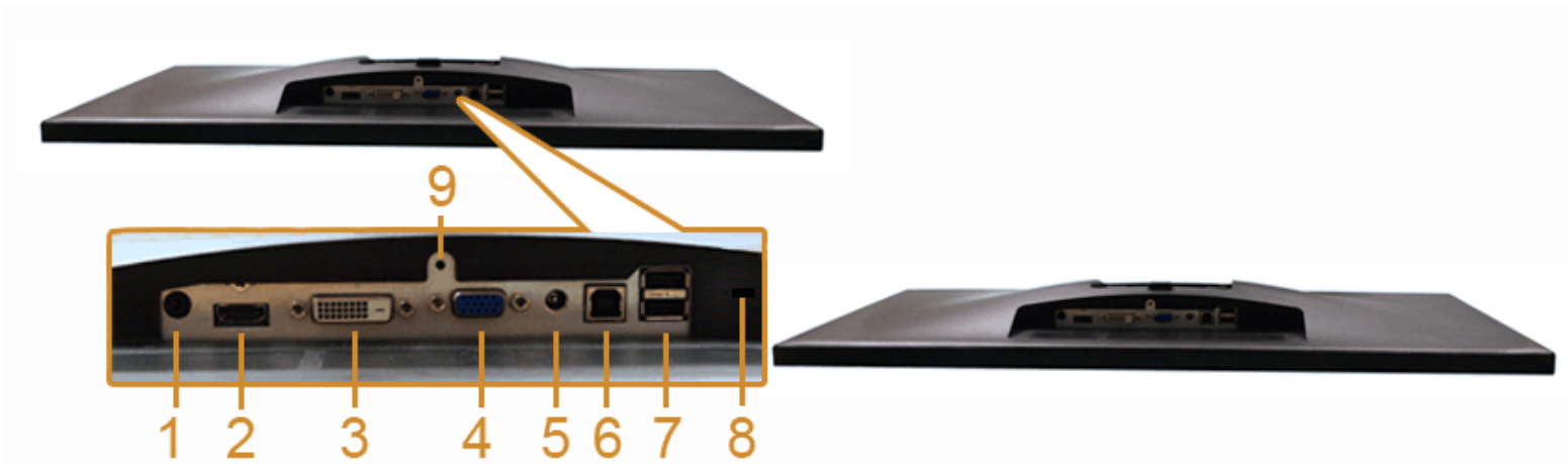
モニタスタンドなし底面図
